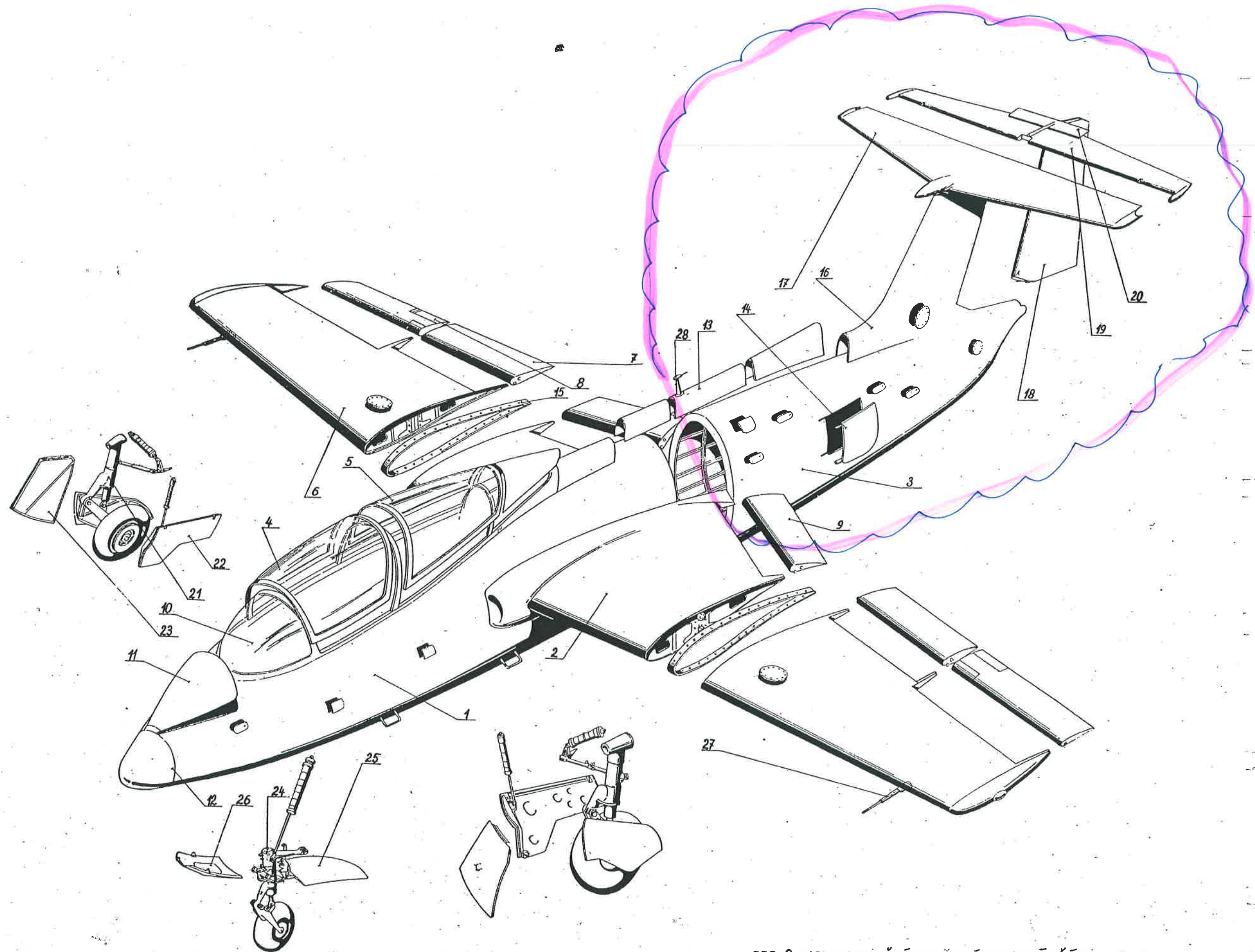
OBR. 2 - KONSTRUKČNÍ A ROZEBÍRATELNÉ ČÁSTI
